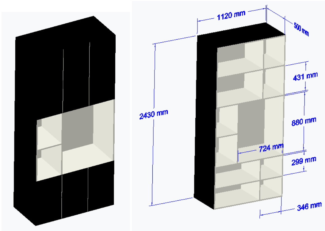
Figura 1: Dimensões e disposição das prateleiras.
